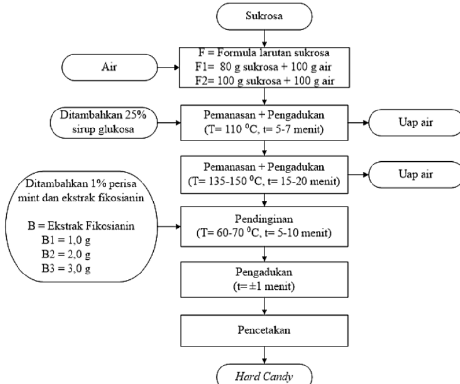
Gambar 2. Diagram Alir Proses Pengolahan Hard Candy (Modifikasi dari Kurnia, 2009)
