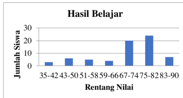
Gambar 1. Diagram Batang Skor Hasil Belajar
