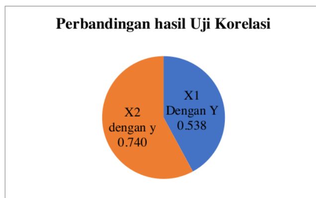
Gambar 2 Perbandingan Hasil Uji Korelasi
