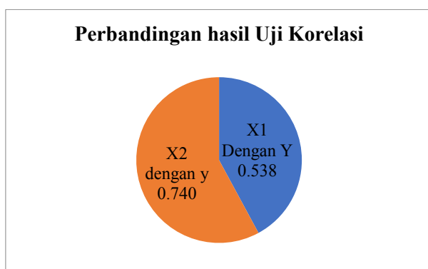
Gambar 2 Perbandingan Hasil Uji Korelasi
