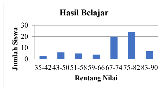
Gambar 1. Diagram Batang Skor Hasil Belajar
